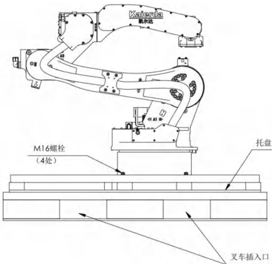
图 2-2: 使用叉车时的搬运方法
