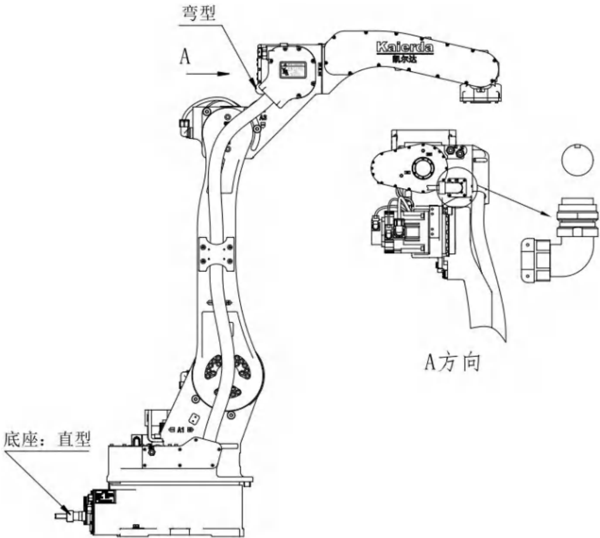
图 7-5: 装备电线连接插头安装图
