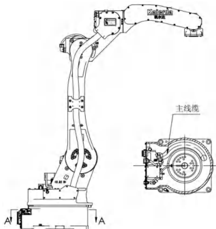
图 7-3: 电线的配置
