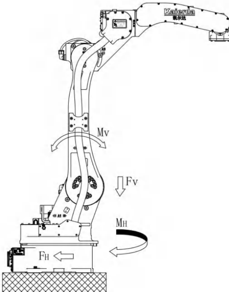
图 3-1: 机器人安装结构反力和力矩
