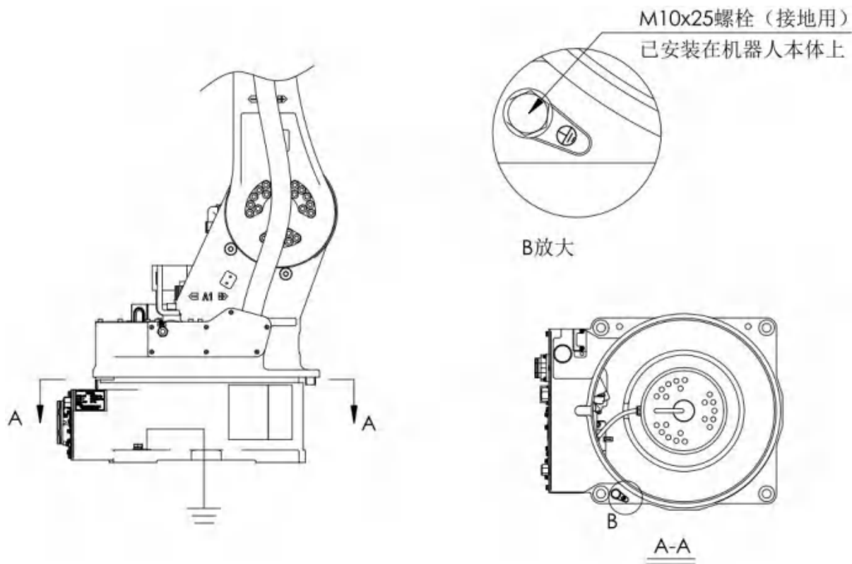
图 4-1: 接地方法
