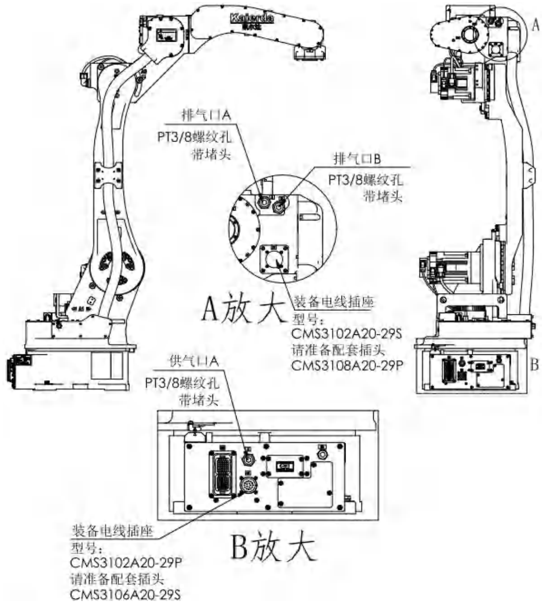
图 7-2: 装备电线和气管
