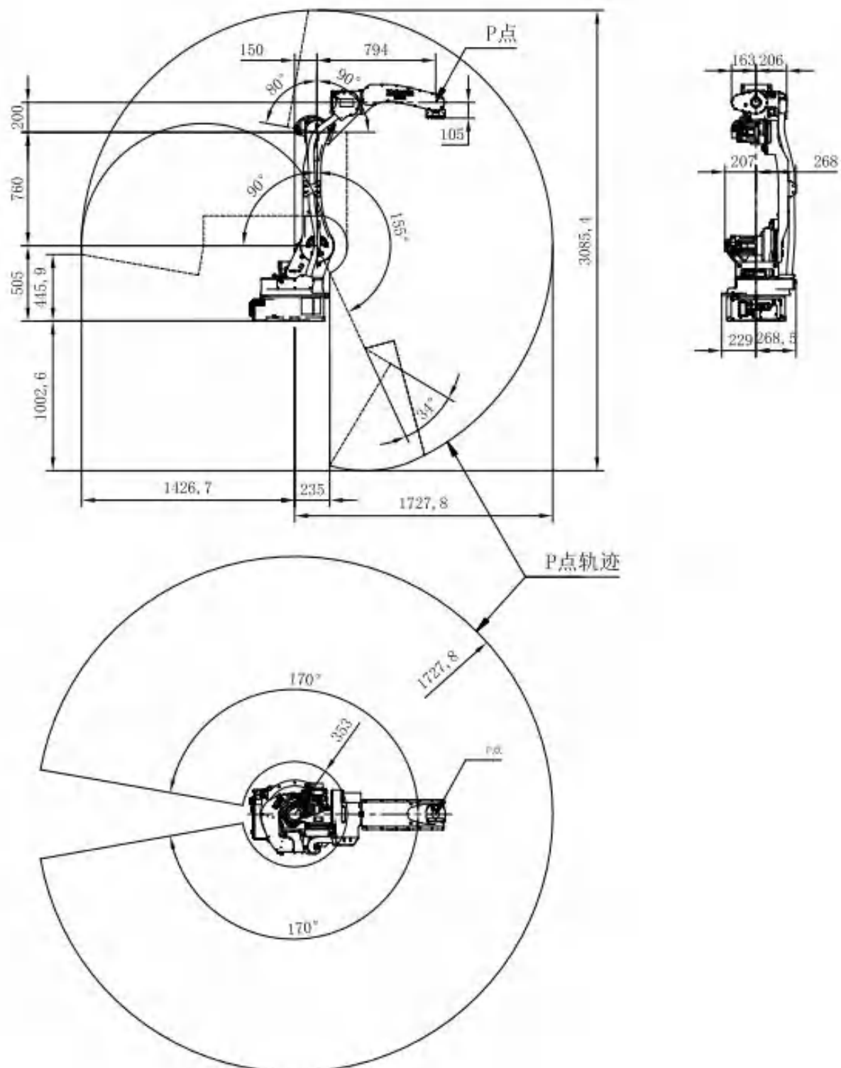
图 5-3: 外形尺寸以及可动范围
