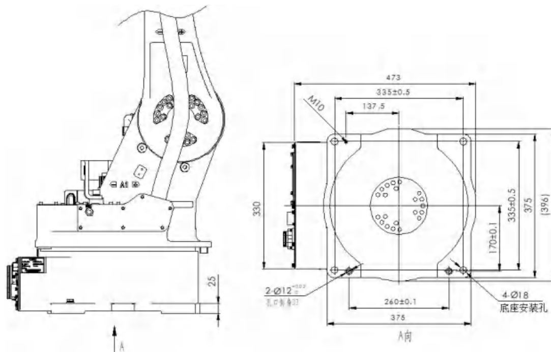
图 5-2: 机器人安装尺寸
