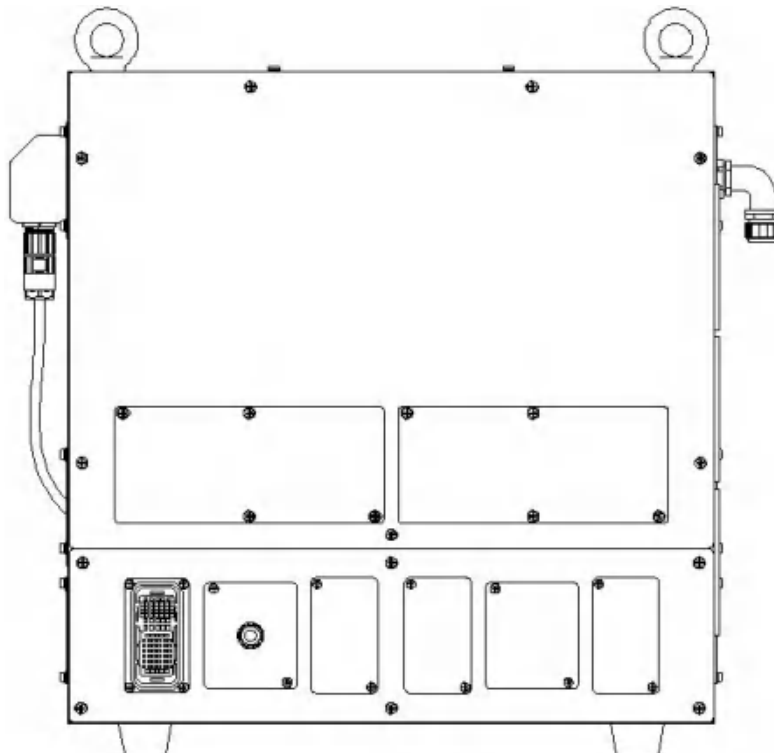
图 4-5: KC30～通讯线缆连接部
