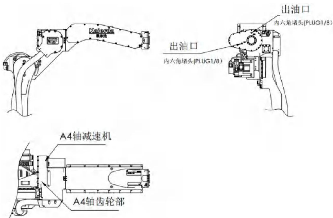
图8-7: A4 轴减速机及齿轮部构造
