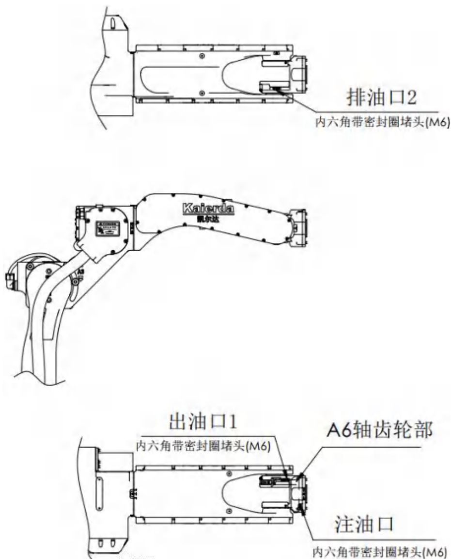
图8-10: A6轴齿轮构造
