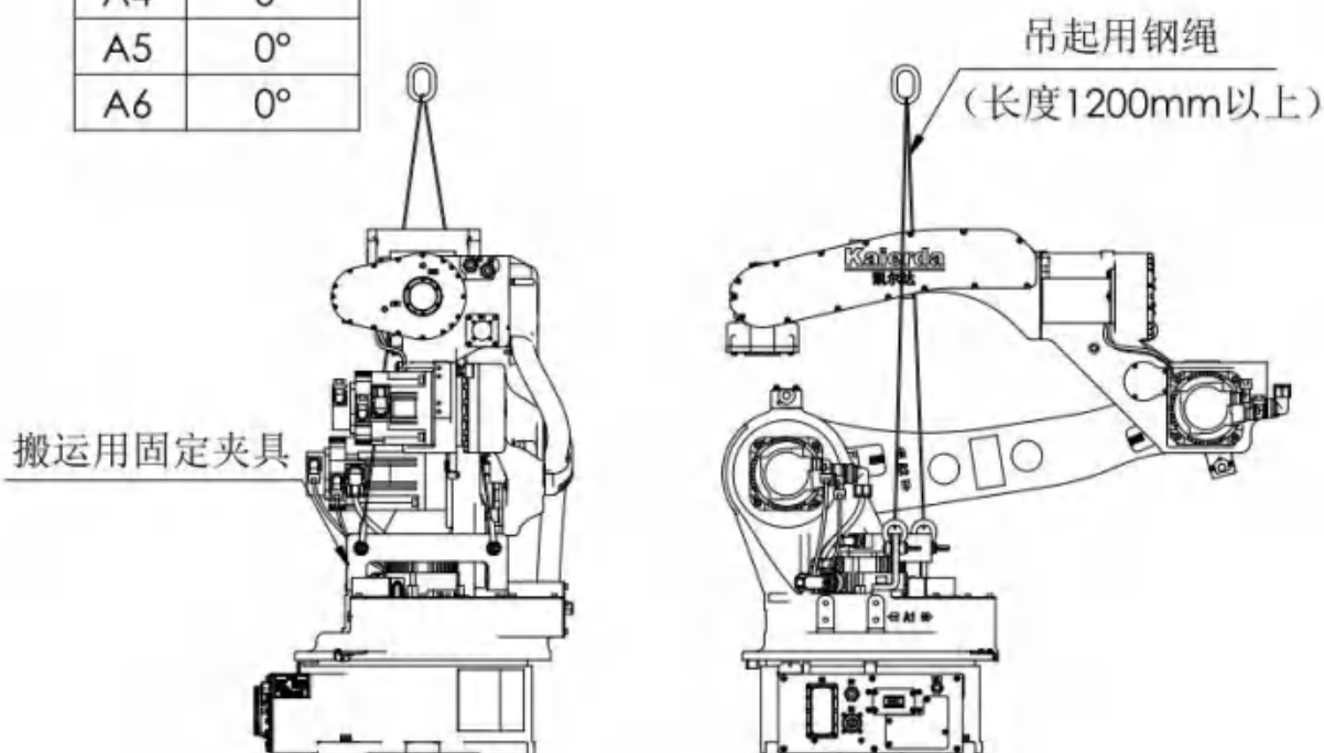
图2-1: 搬运姿势
