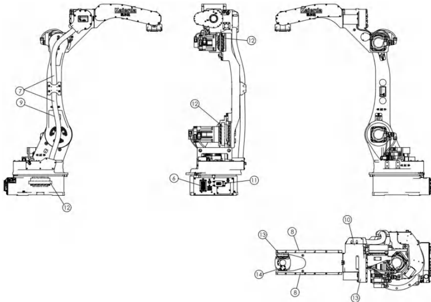
图 8-1: 检修位置与作业编号 (原点姿势图)
