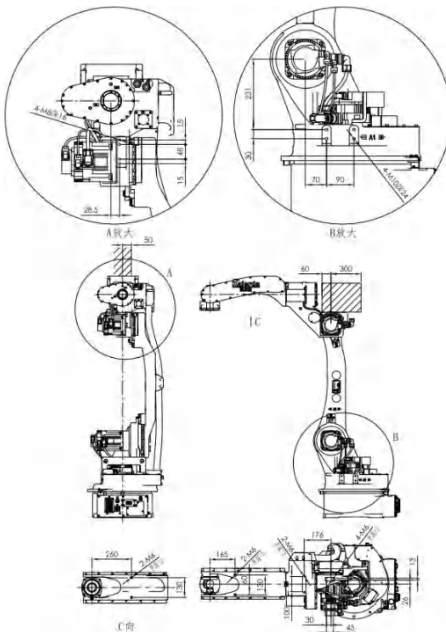
图7-1: 安装底座
