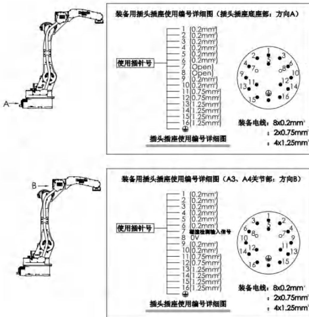
图 7-4: 插头插座号码的详细介绍
