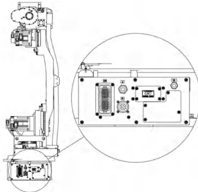
图 4-4: KP25本体～通讯线缆连接部
