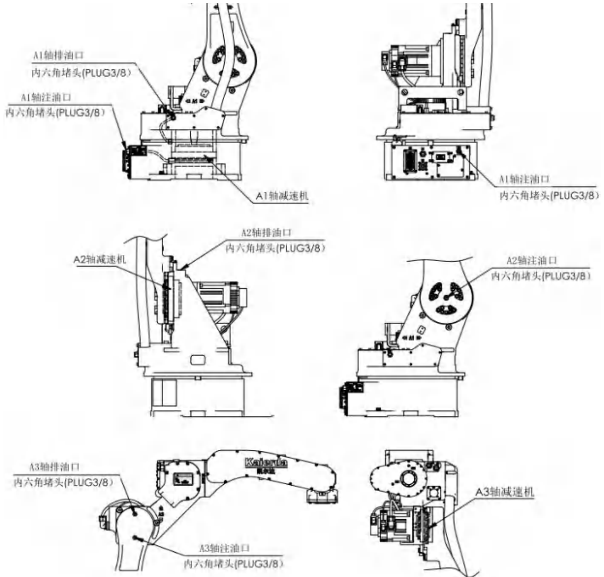
图 8-5: A1.A2.A3 轴减速机构造
