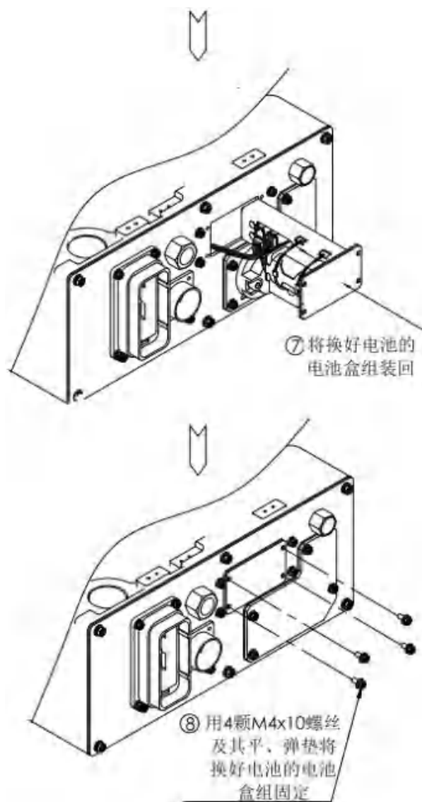
图 8-2: 电池组更换步骤
