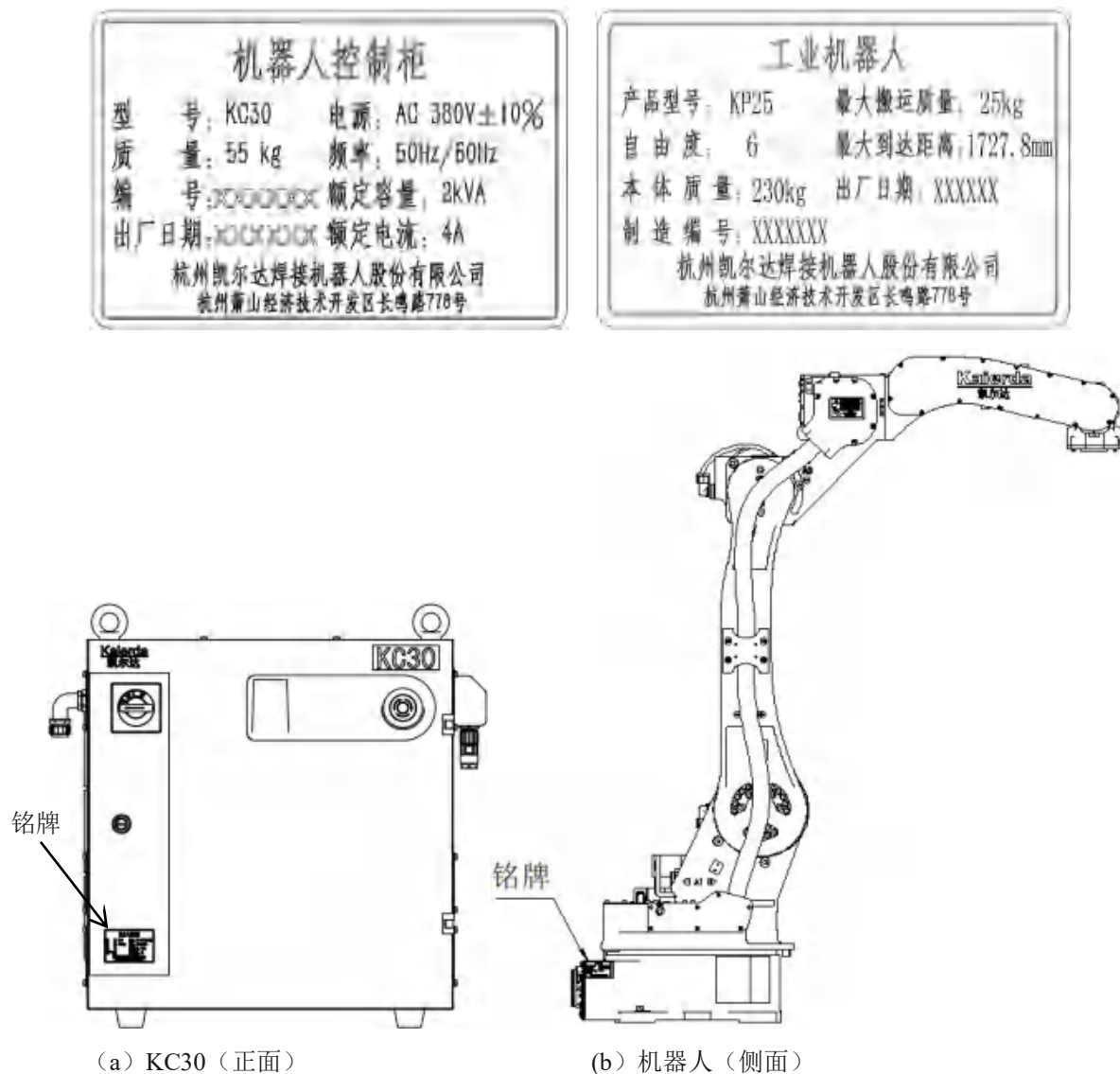
图 1-2: 铭牌的粘贴位置
