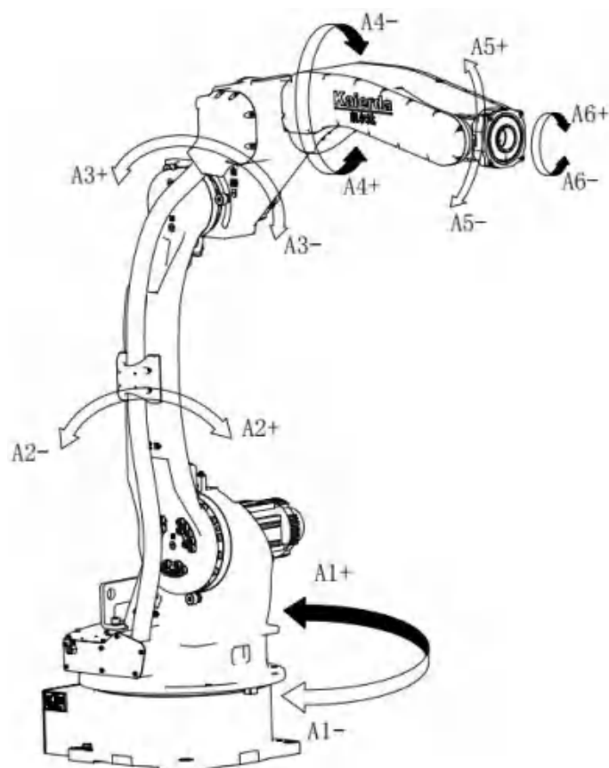
图 5-1: 机器人各部位和各轴名称
