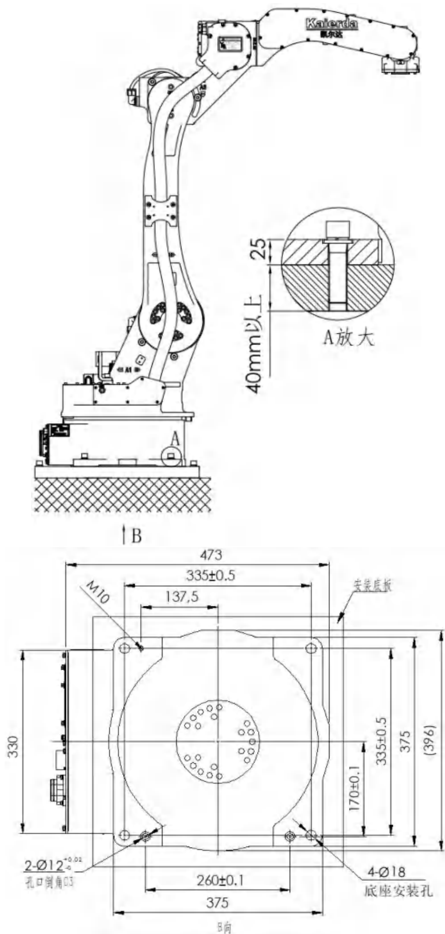
图 3-2: 机器人安装案例
